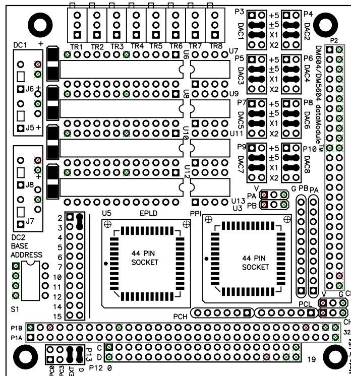
Fig. 5-1 — Module Layout
